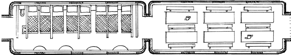
QUARTIERS DE L'ÉQUIPAGE
